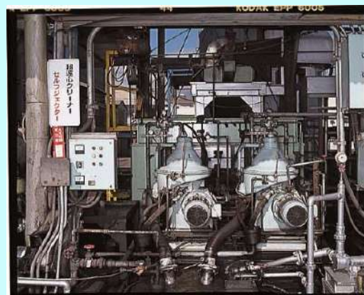
遠心分離施設（再生重油）
